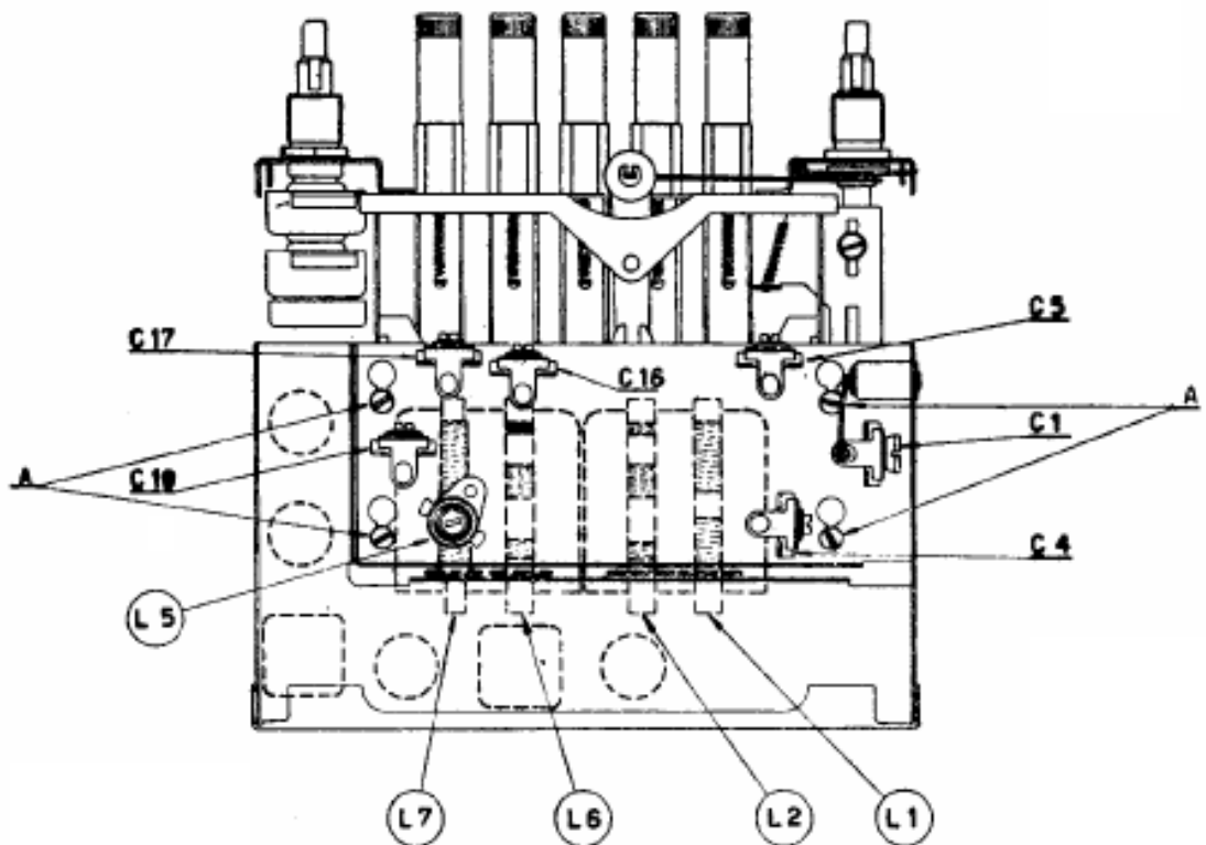
AUTOVOX RA 23 - Posizione degli organi di taratura.
